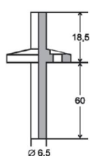
Kanalanschlussnippel 6551
