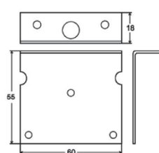
Befestigungswinkel Typ 6401
