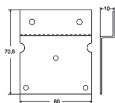
Befestigungswinkel Typ 6402
