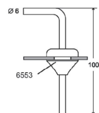
Kanalanschlussnippel 6552 mit Gummidurchführung 6553
